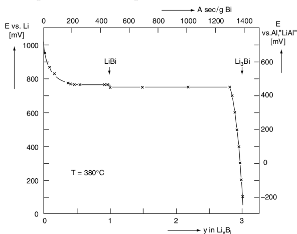
FIGURE 9 – Évolution de la f.e.m. de la pile lors d'un titrage coulométrique d'une pile Li-Bi menée à 380^\circ\text{C}
