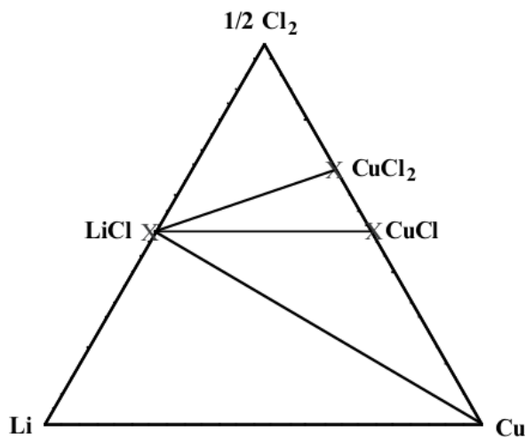
FIGURE 12 – Diagramme ternaire isotherme à 25 °C où les corps purs, simples et complexes, sont indiqués
