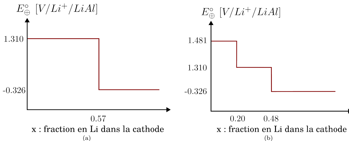
FIGURE 16 – Évolution de la force électromotrice par rapport à la référence \text{Li}^+/\text{LiAl} à 400^\circ\text{C} 16a dans le cas d'un pôle \oplus constitué à l'état chargé d'une phase \text{LiCoO}_2 ; 16b dans le cas d'un pôle \oplus constitué à l'état chargé d'une phase \text{CoO} .
