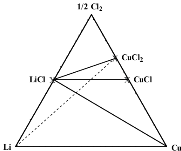
FIGURE 14 – Ligne de composition lorsque la fraction de lithium varie au sein d'une pile \text{Li}||\text{CuCl}_2
