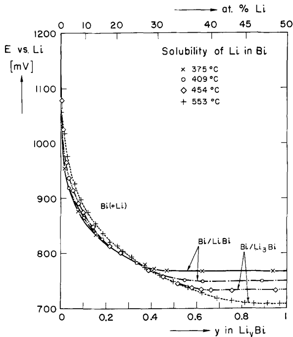
FIGURE 10 – Évolution de la force électromotrice de la pile Li||Bi à différentes températures, zoomé sur l'écart au modèle initial dans le domaine de stoechiométrie 0 < x < 1
