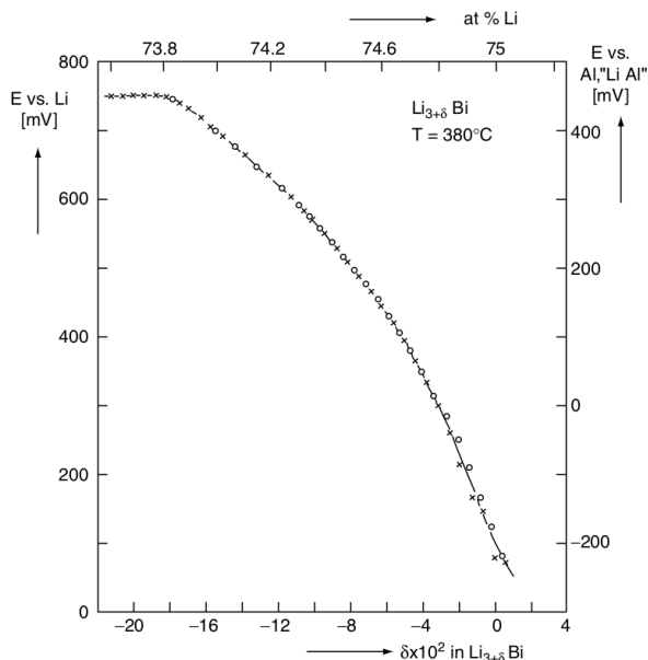
FIGURE 11 – Évolution de la force électromotrice de la pile \text{Li}||\text{Bi} à 380^\circ\text{C} , zoomé sur l'écart au modèle initial dans le domaine proche du composé défini " \text{Li}_3\text{Bi} "
