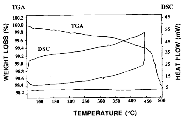
FIGURE 23 – Analyse par thermogravimétrie et par analyse calorimétrique différentielle de la phase délithié \text{FePO}_4 en présence d'une atmosphère inerte (diazote).
