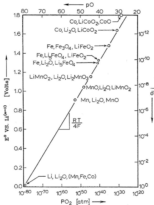
FIGURE 17 – Évolution du potentiel du pôle \oplus composés de systèmes ternaires lithiés en fonction de la pression d'équilibre tirée des diagrammes d'Ellingham des oxydes non lithiés.
