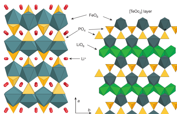
FIGURE 22 – Structure de l'olivine \text{LiFePO}_4 dans la projection le long de [001].
