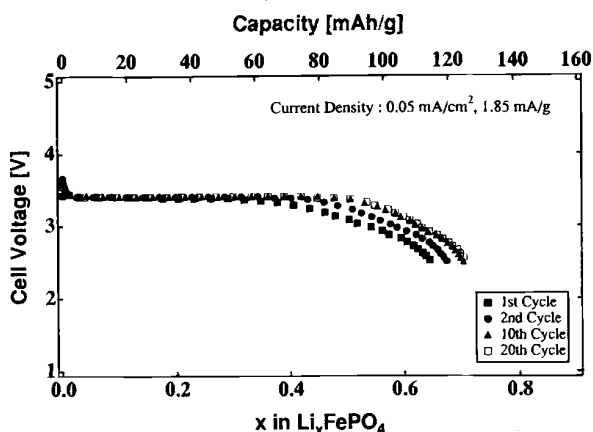
FIGURE 24 – Évolution du potentiel cathodique par rapport à une électrode au lithium pour une densité de courant de 0.05 mA en fonction de la fraction en lithium dans \text{Li}_x\text{FePO}_4 .
