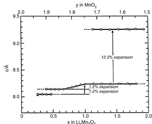
FIGURE 21 – Évolution du paramètre de maille en fonction de la stoechiométrie en lithium dans \text{Li}_x \text{Mn}_2 \text{O}_4 .
