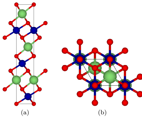
FIGURE 19 – 19a Maille conventionnelle du composé de stœchiométrie \text{Li}_3\text{Co}_3\text{O}_6 projetée le long de [100] . 19b Maille conventionnelle du composé de stœchiométrie \text{Li}_3\text{Co}_3\text{O}_6 projetée le long de [001] .
