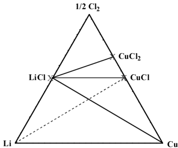
FIGURE 13 – Ligne de composition lorsque la fraction de lithium varie au sein d'une pile \text{Li}||\text{CuCl}
